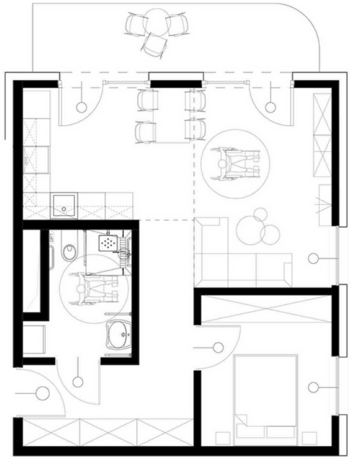
LOKALIZACJA MIESZKANIA TYPU I NP
