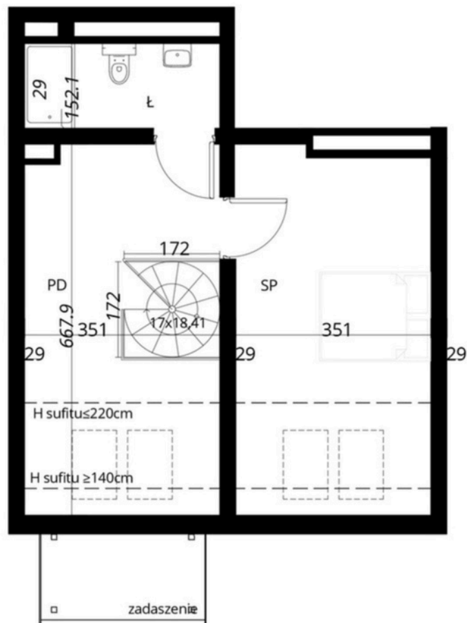
LOKALIZACJA MIESZKANIA TYPU 10 I PIĘTRO
