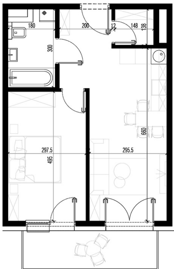
LOKALIZACJA MIESZKANIA TYPU I
