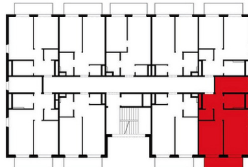
LOKALIZACJA MIESZKANIA TYPU VIII
